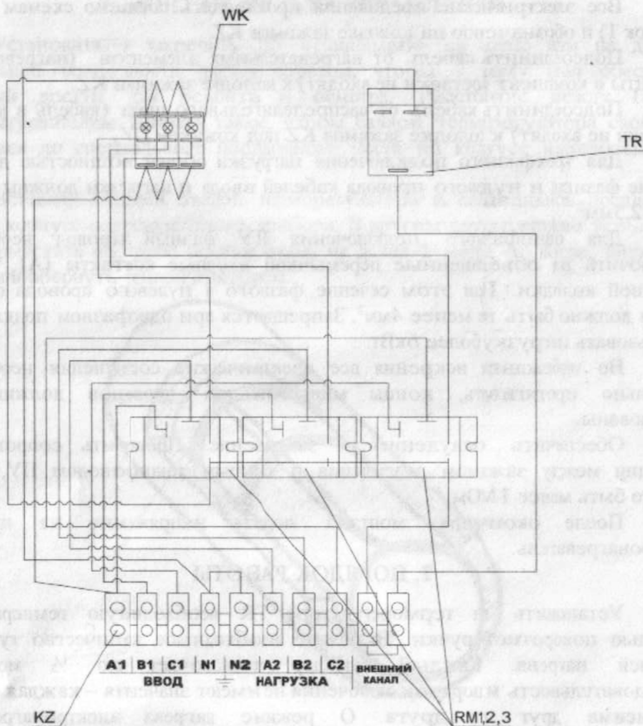
Рис.2 Схема монтажная.
