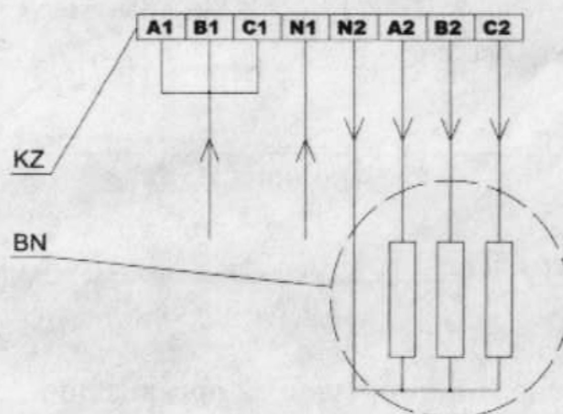
Рис. 1б Пример однофазного подключения ТЭНБ-6
