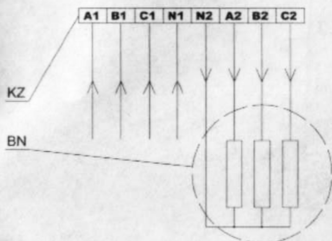
Рис. 1а Пример трехфазного подключения ТЭНБ-6, ТЭНБ-9
