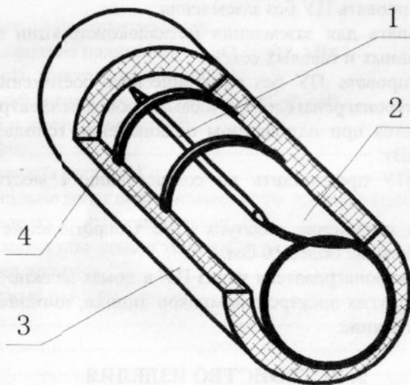
Схема установки датчика терморегулятора.
