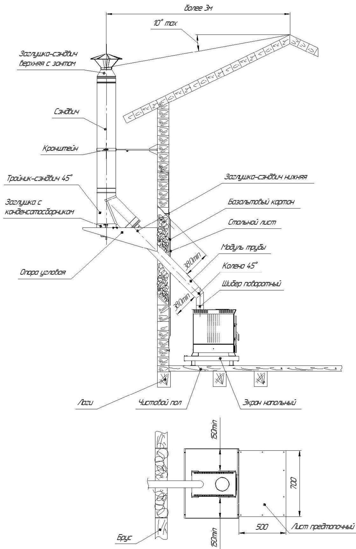
Рисунок 6 - Рекомендуемая схема установки печи
