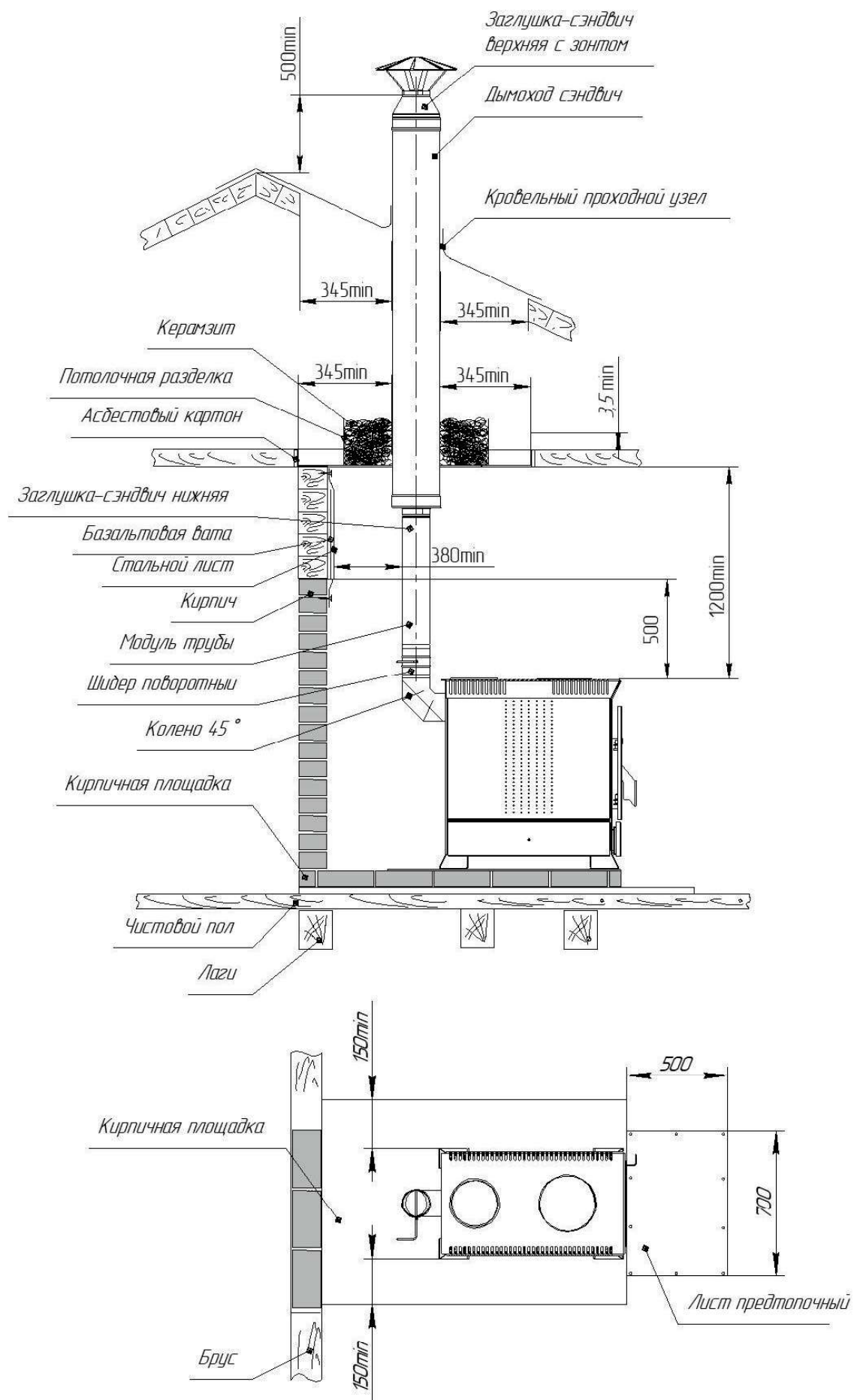
Рисунок 4 - Рекомендуемая схема установки печи
