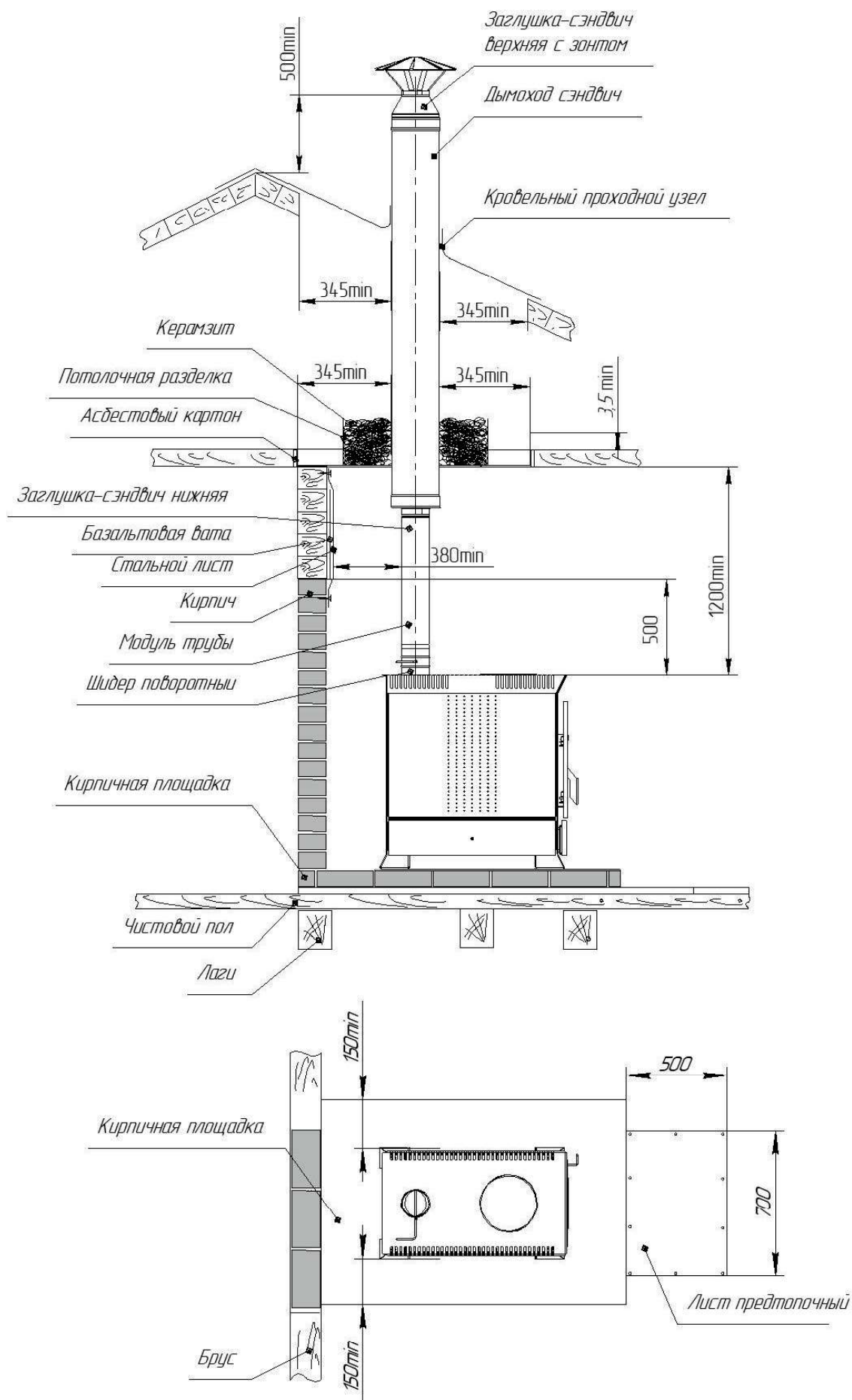
Рисунок 5 - Рекомендуемая схема установки печи
